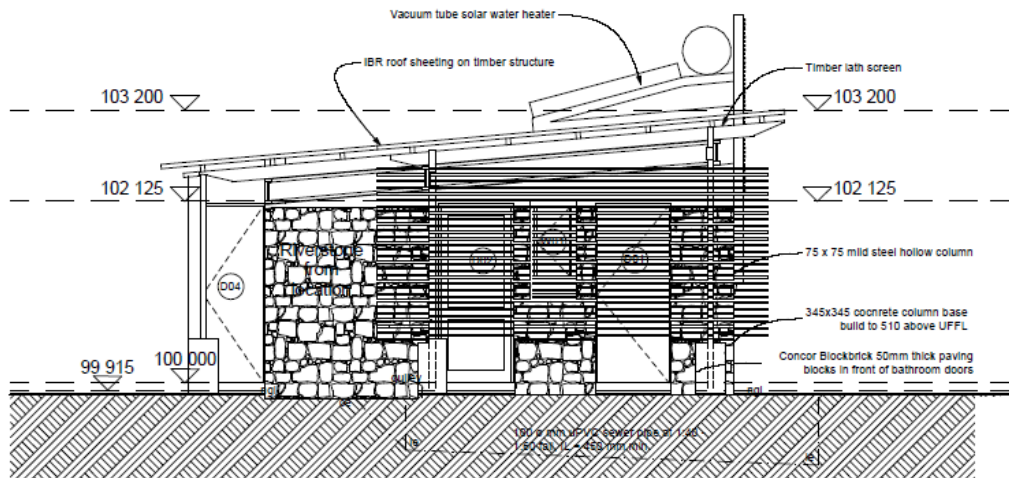
West Elevation Scale: 1:50
