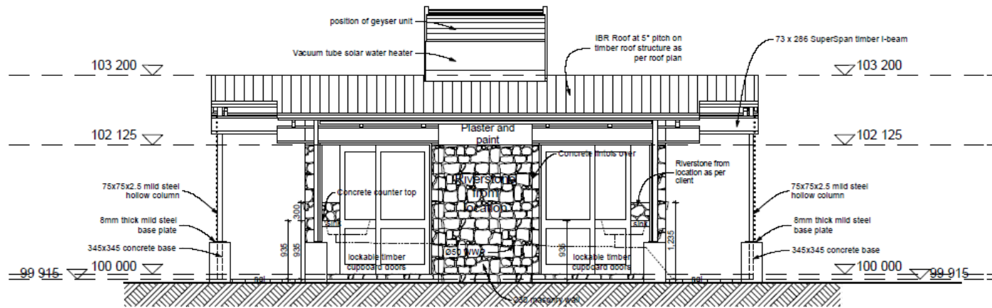
North Elevation Scale: 1:50
