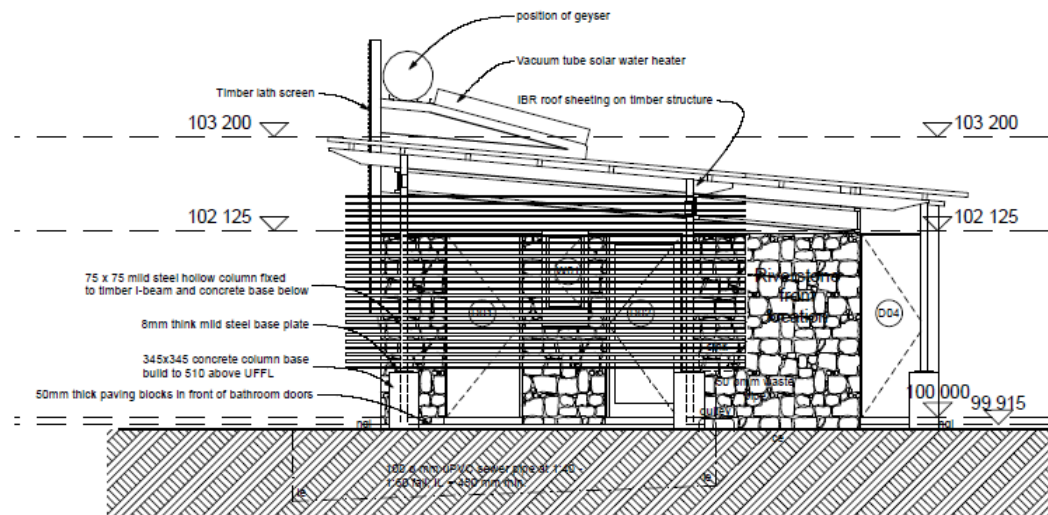
East Elevation Scale: 1:50
