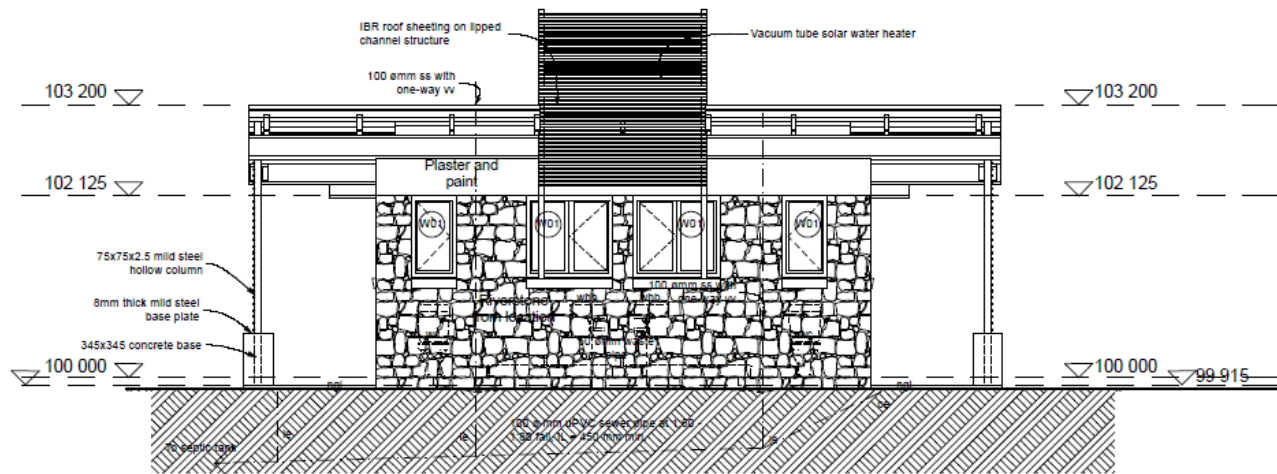
South Elevation Scale: 1:50
